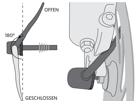
Abb. 1. Schnellspanner öffnet sich mehr als 180 Grad
